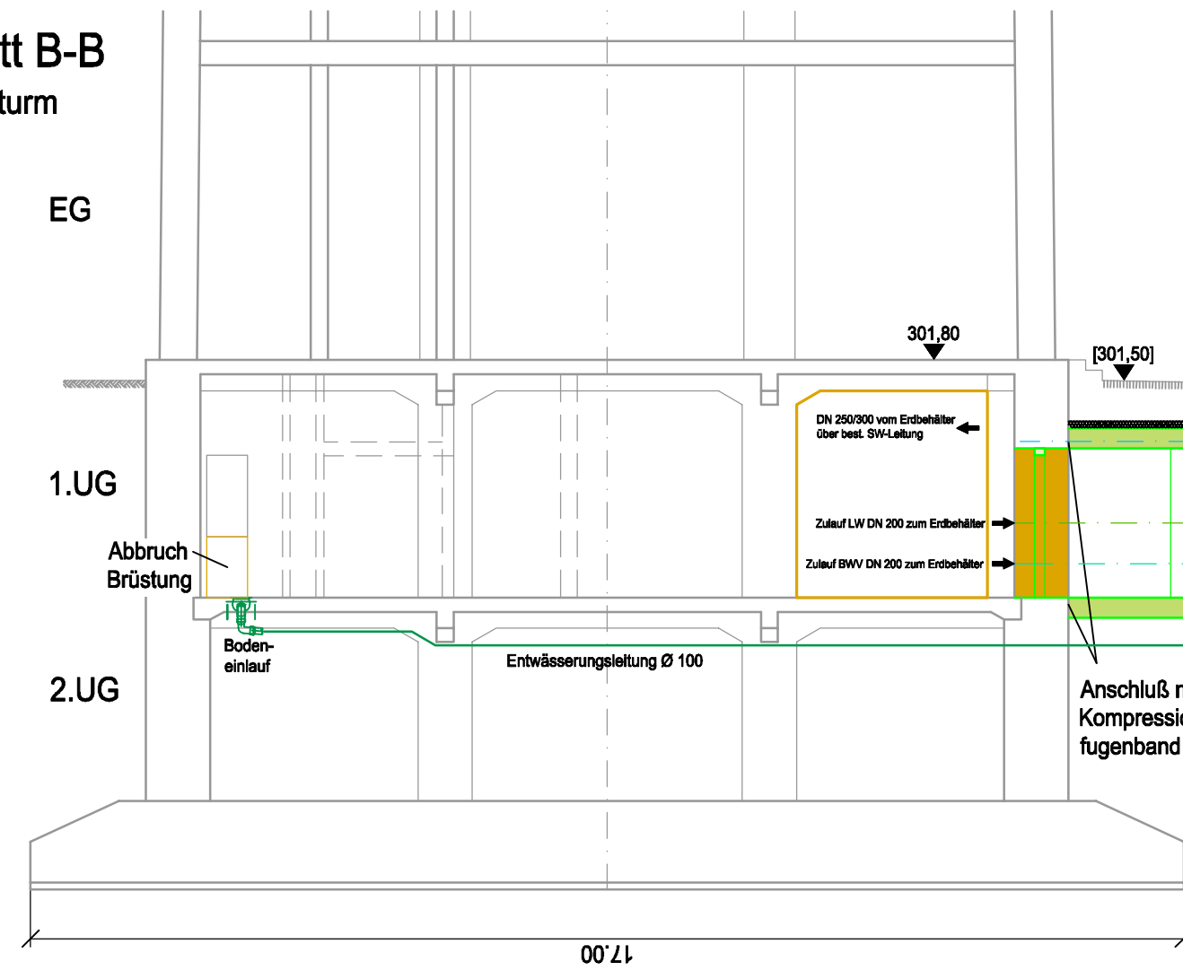
1. Untergeschoß Wasserturm
