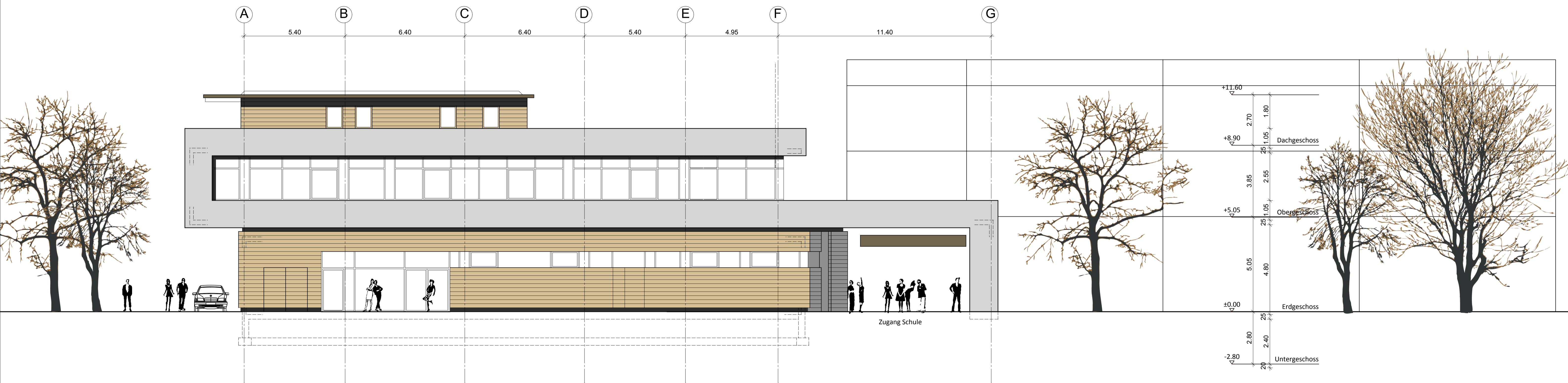
Ansicht Ost
