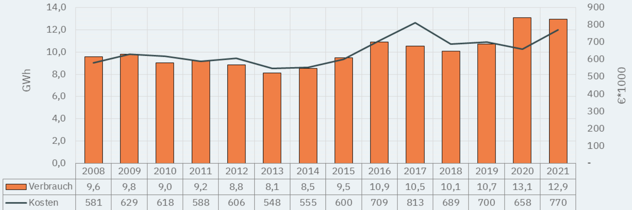
Wärmeverbrauch - witterungsbereinigt
